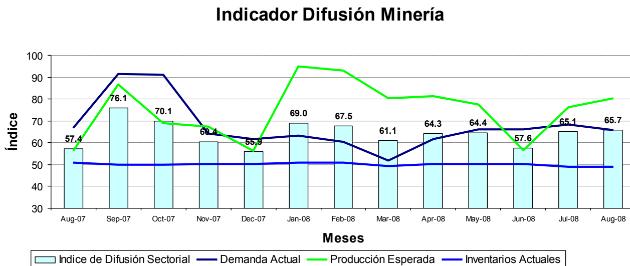
Figura 8. Indicador Difusión del Sector Minería
