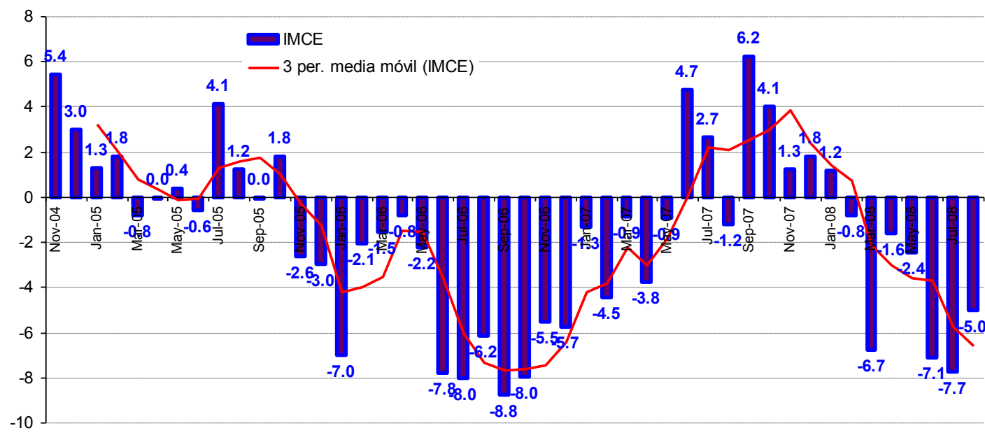
Figura 1c. Variación del IMCE en 12 Meses y Velocidad medida por su Media Móvil de tres Meses
